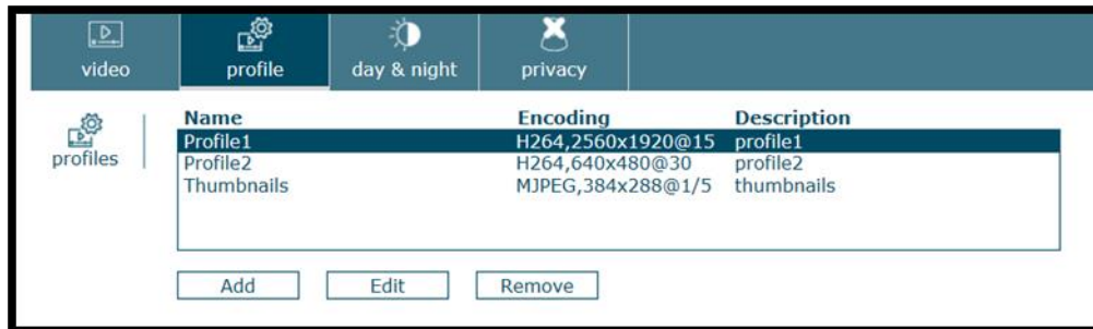
圖 9. 新增/編輯碼流設定檔頁面
