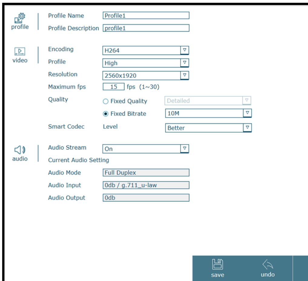
圖 9. 新增/編輯碼流設定檔頁面
